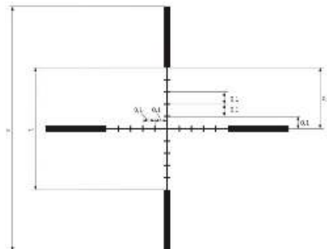
Рисунок 33 – Прицельная сетка (размер в м/100м дистанции)
