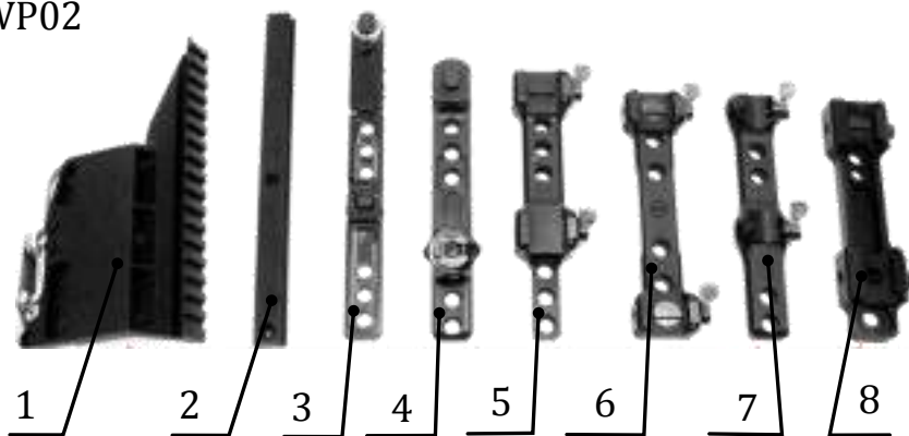
Рисунок 31 – Планки крепления к оружию
