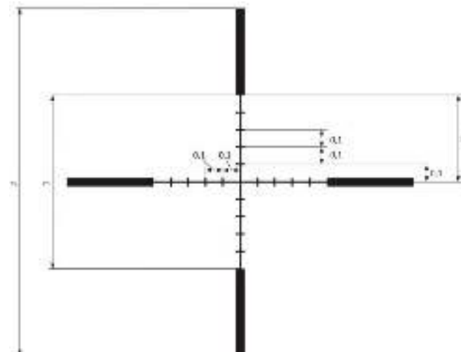
Рисунок 32 – Прицельная сетка (размер в м/100м дистанции)
